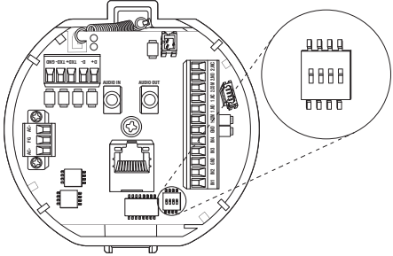
通信プロトコルのDIPスイッチ（SW1）
