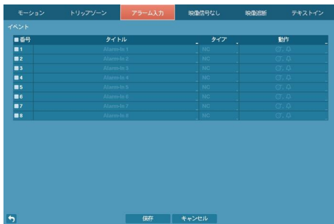
図 20: イベント→アラーム入力設定画面
