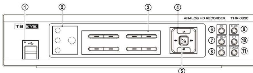
図 3: DVR前面パネル
