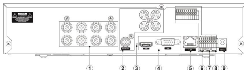
図 2: DVR背面パネル
